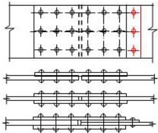
Hình 2.32: Liên kết đối đầu dùng bán ghép
