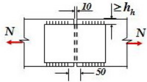
Hình 2.24: -Lk đối đầu dùng đh góc cạnh
