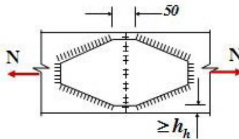
Hình 2.27: Liên kết hỗn hợp
