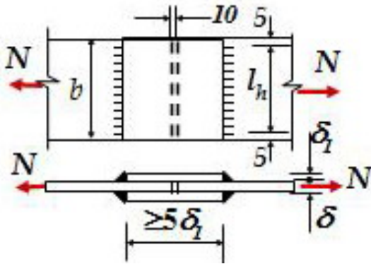
Hình 2.23: -Lk đối đầu dùng đh góc đầu
