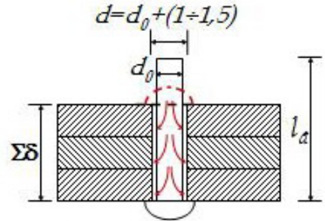
Hình 2.28: Liên kết đinh tán
