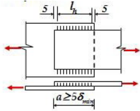
Hình 2.20: Lk chồng dùng đh góc cạnh
