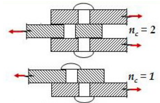
Hình 2.37: Khả năng chịu cắt của đinh tán
